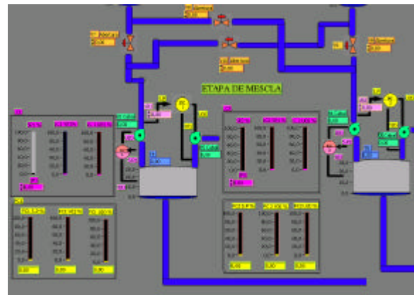
Figura 6: Sistema SCADA: Etapa de mezcla.
